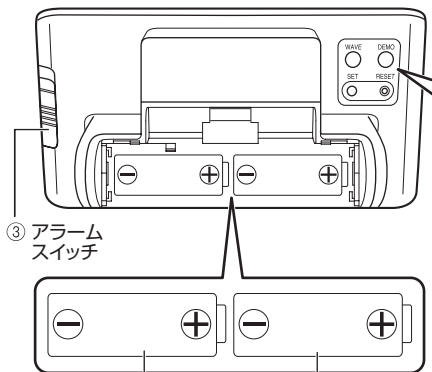
単2形アルカリ乾電池(LR14)×2
